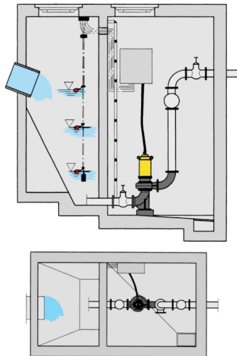
Рис. 6. Ejecución IS: instalación en seco / IS configuration: dry pit installation / IS-установка: Сухая установка
