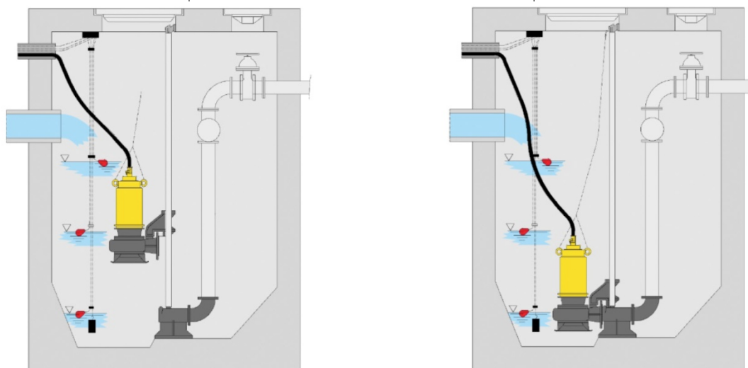
Рис. 7 Ejecución IP: instalación en pozo colector, con dispositivo de amarre rápido
