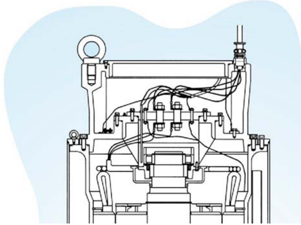
Рис. 2. Caja de conexiones / Terminal box / Клеммная коробка
