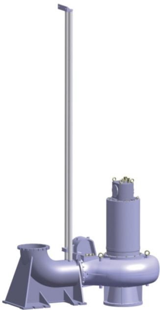
a- Instalación: en pozo húmedo (dispositivo de amarre rápido) a-Wet pit installation (quick coupling type) a- «Мокрая» стационарная установка (быстроразъемное соединение)
