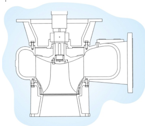
Рис. 4. Partes hidráulicas / Hydraulic parts / Улитка (Корпус насоса)
