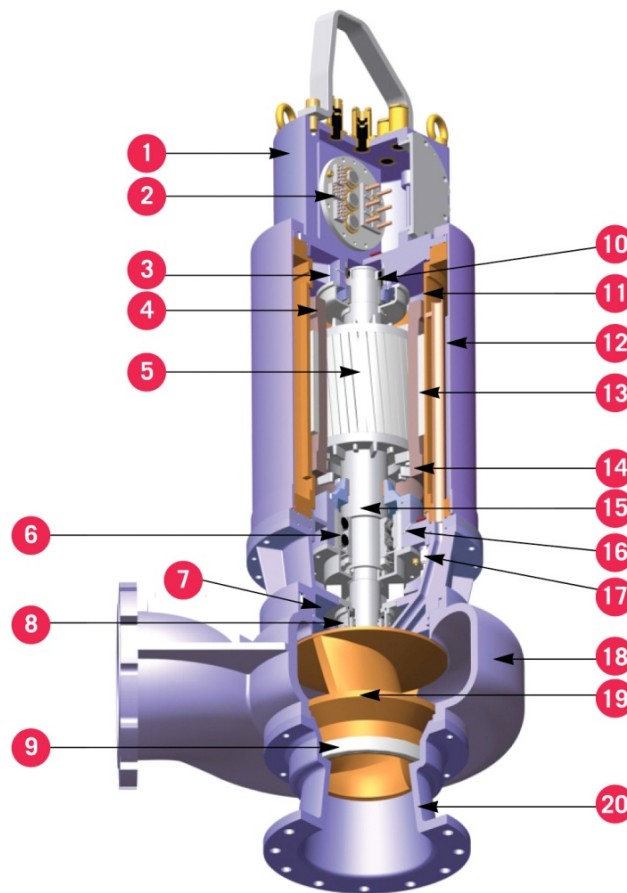
Рис. 1. Vista seccional del grupo / Cross section of a pumping set / Разрез насосного агрегата.
